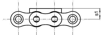
WA-2 unašeč (jedostranný)
