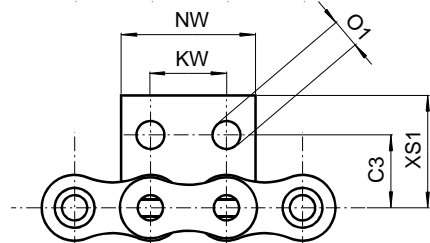
WSA-2 unašeč (jedostranný)
