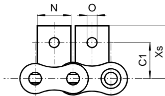
SA-1 unašeč (jedostranný)
