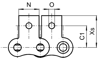
SK-1 unašeč (oboustranný)
