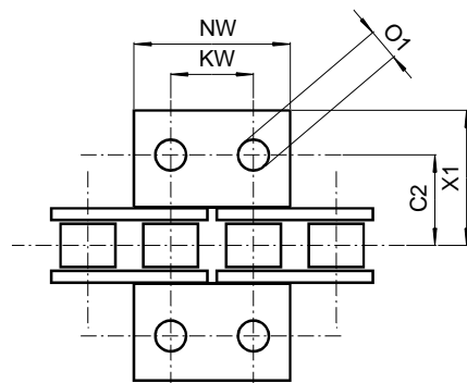
K-1 unašeč (oboustranný)
