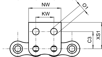
WSK-2 unašeč (oboustranný)
