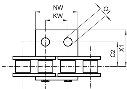
A-1 unašeč (jedostranný)
